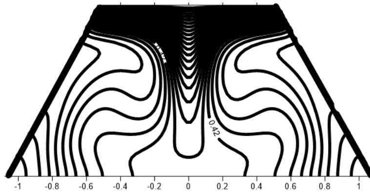
Fig. 7. Distribution of moisture isovalues contours for Pr=0.71 ; F=1 ; Ra=7.10^2
