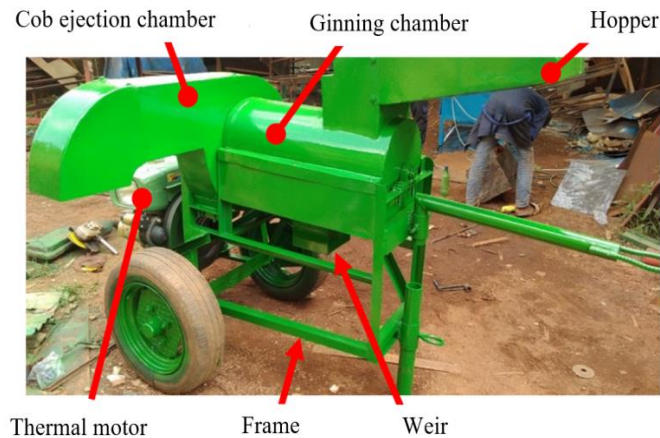
Fig. 1. ZEKEDA maize sheller
