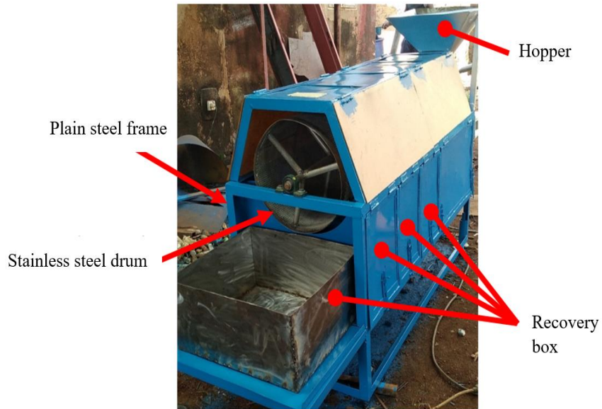
Fig. 9. Flour roller
