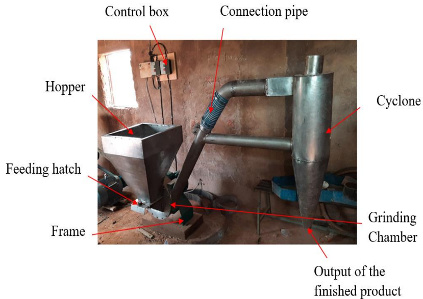
Fig. 8. Hammer mill
