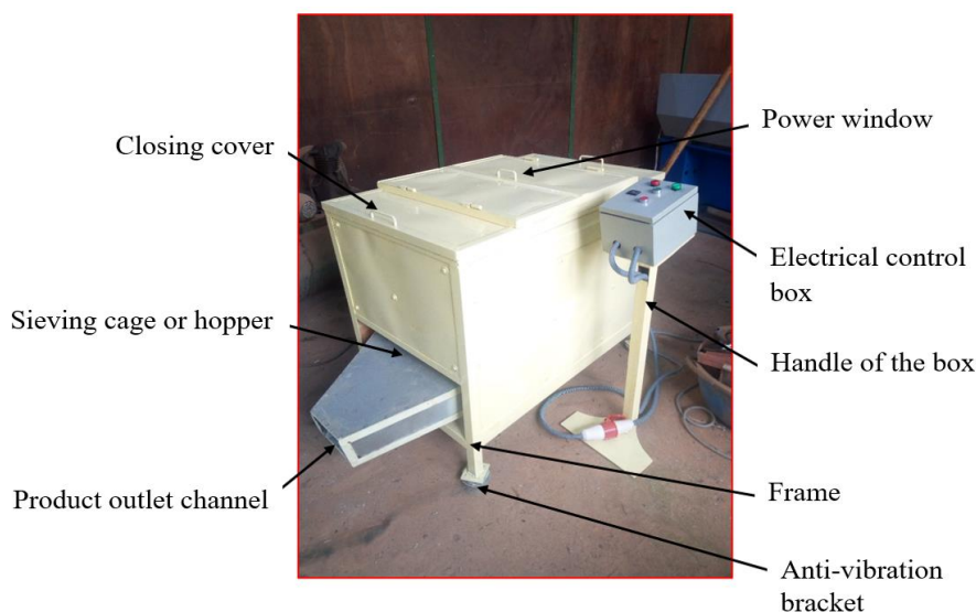
Fig. 12. The flour sieve
