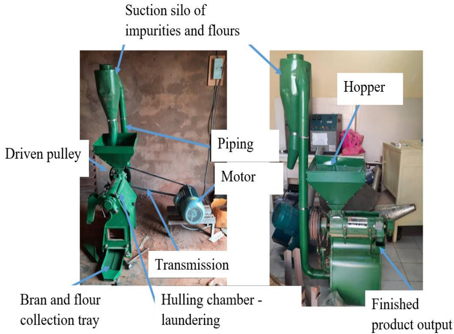
Fig. 7. Cereal husker
